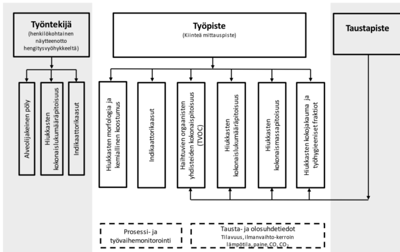
Kuva 8. Työpaikamittauksissa käytetty mittausjärjestely.
