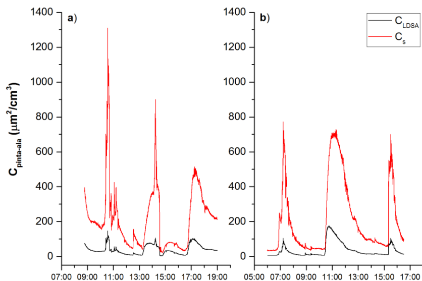
Kuva 24. DiSCmini:n mitaamat hiukkasten kokonaispinta-alapitoisuuden ( C_s ) ja keuhkojen alveolialueelle teoreettisesti deponoituvien hiukkasten pitoisuuden ( C_{LDSA} ) aikasarjat kampaamossa työpisteessä a) ensimmäisenä mittauspäivänä, b) toisena mittauspäivänä.
