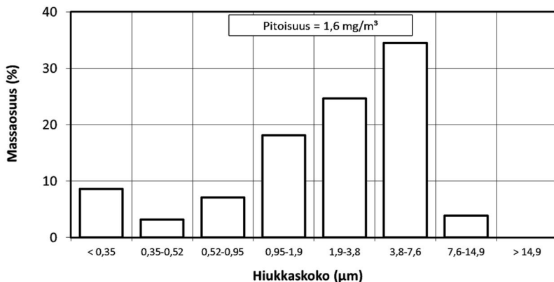
Suodatinyksikkö 5
