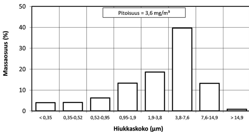
Suodatinyksikkö 1-a
