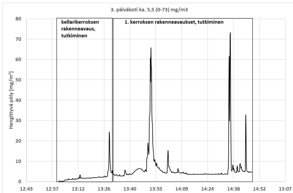
Kuva 13. Hengittyvän pölyn pitoisuusvaihtelu asiantuntijan hengitysvyöhykkeellä kohteessa 3.
