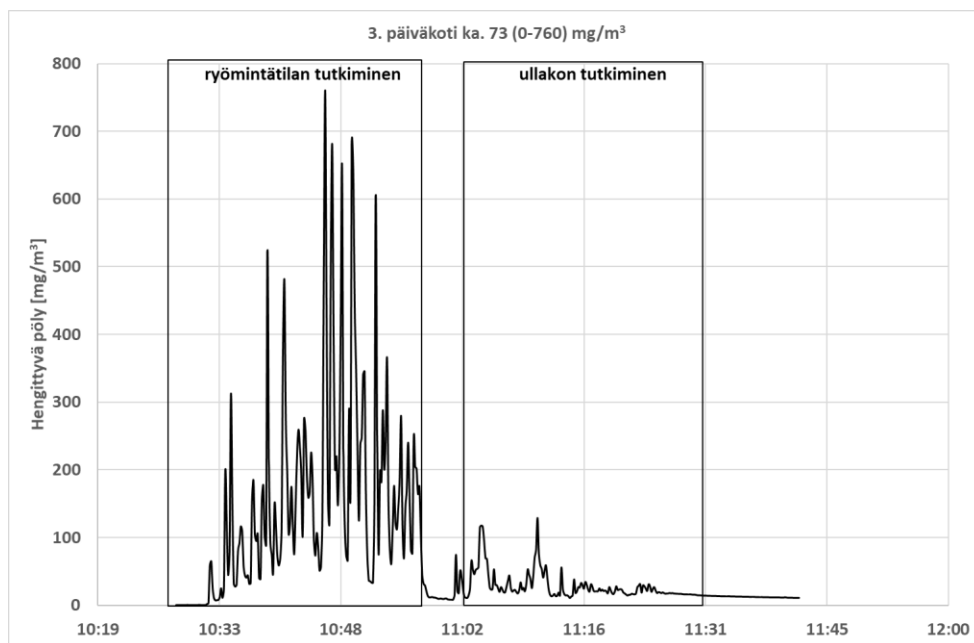
Kuva 12. Hengittyvän pölyn pitoisuusvaihtelu asiantuntijan hengitysvyöhykkeellä kohteessa 3
