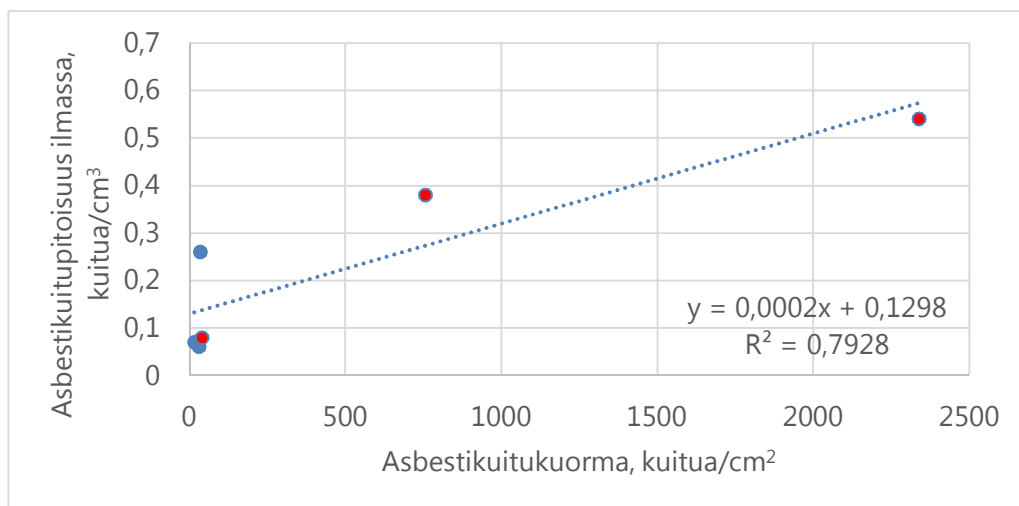
Kuva 9. Työtakkien keskimääräisen asbestikuitu-altistuksen korrelaatio takista imuroituun asbestikuitukuormaan nähden; rikastamon prosessimiesten altistamat (punainen) ja tutkijoiden altistamat (sininen)
